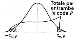
Tavola A3 - Percentili della distribuzione t - La funzione tabulata è t_{v,P} valore superato in entrambe le direzioni con probabilità P in una distribuzione t con \nu gradi di libertà
